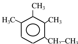
1-etil-2,3,4-tri- metilbenceno
