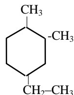
4-etil-1,2-dimetil- ciclohexano
