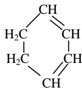
1,3-ciclohexadieno
