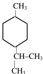
1-metil-4-isopro- pilciclohexano
