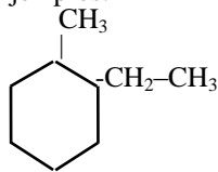
1-etil-2-metil- ciclohexano
