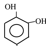
1,2,4-trihidroxibenceno
