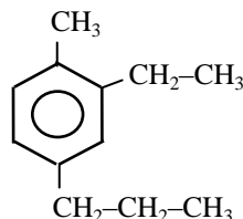
2-etil-1-metil-4-pro- pilbenceno
