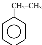
Etilbenceno.
