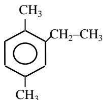
2-etil-1,4-dime- tilbenceno
