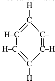
fenilo
